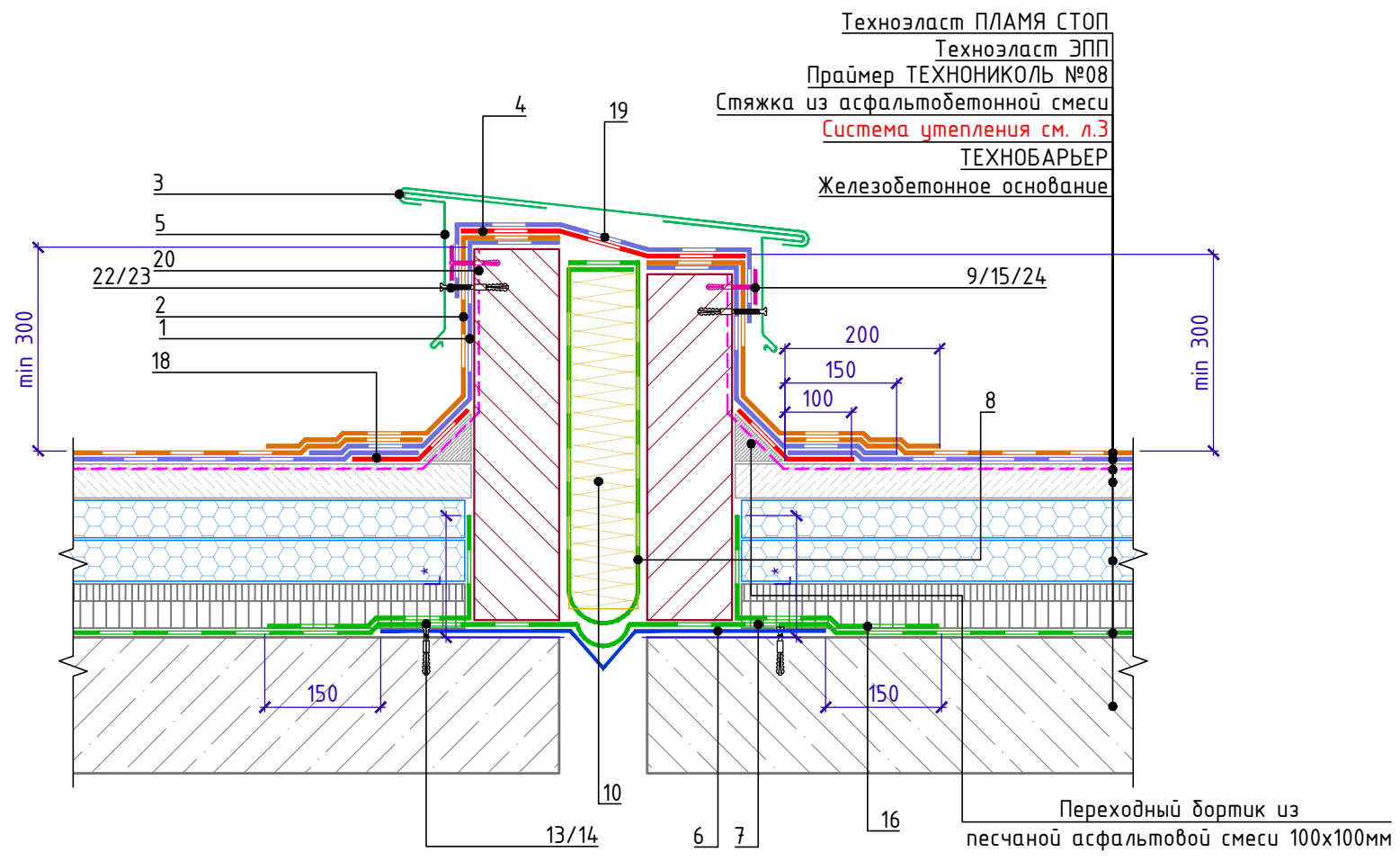
Деформационный разделитель. Вариант 2.
