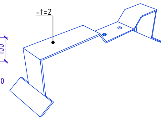
Позиция 8. Схемагиба
